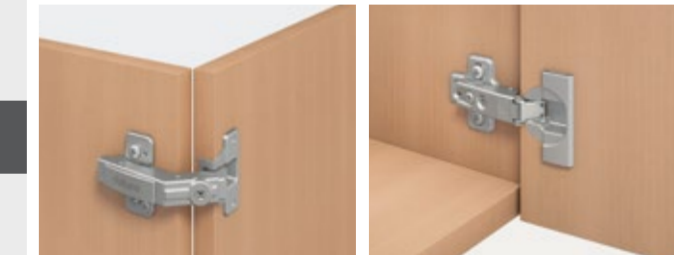
Application pour meuble d'angle Charnières 60° pour meuble d'angle avec porte pliante en combinaison avec la charnière grand angle 155° Application pour réfrigérateur Charnière pour réfrigérateurs avec portes entraînées
